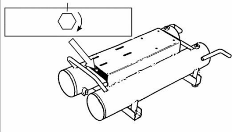
Figura 4 Girar el perno 1/2 pulgada en el sentido de las manecillas del reloj aumentará la tensión de la correa
