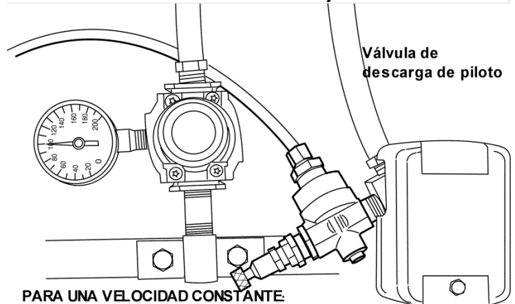
Figura 2 PARA ARRANCAR/APAGAR: Gire el tornillo manual completamente en el sentido de las manecillas del reloj.
